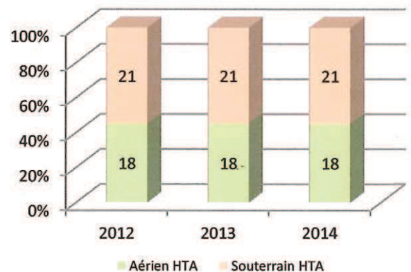
Evolution du réseau haute tension
