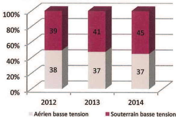
Evolution du réseau basse tension
